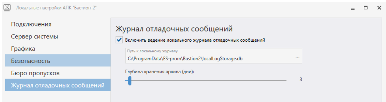
Рис. 77. Настройки логирования
